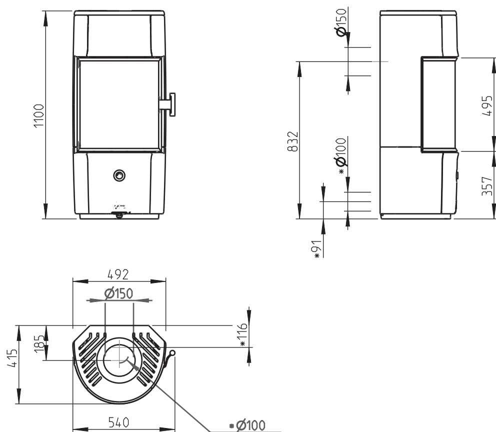
Jøtul F 171 Zensoric
